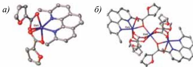
Рис. 1. Молекулярные структуры 1 (а) и 2 (б).
